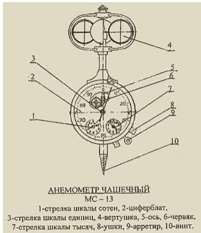
Рис. 1 Чашечный анемометр
