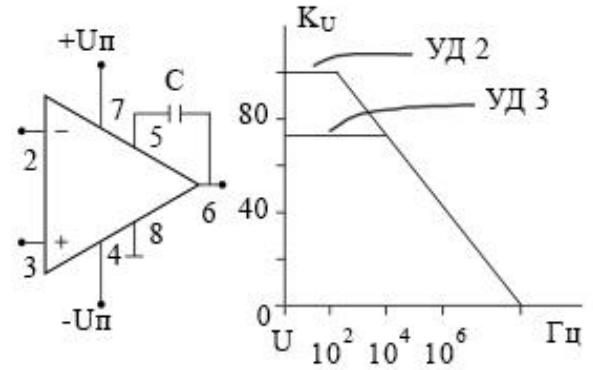
K154УД2 K154УД3
