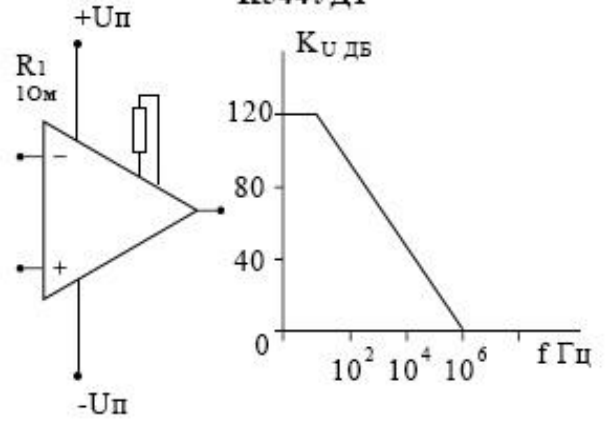
K544УД1
