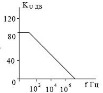
К140УД10
