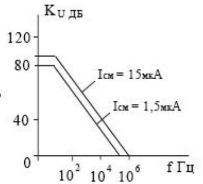
К140УД12
