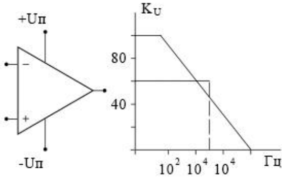
K154УД1
