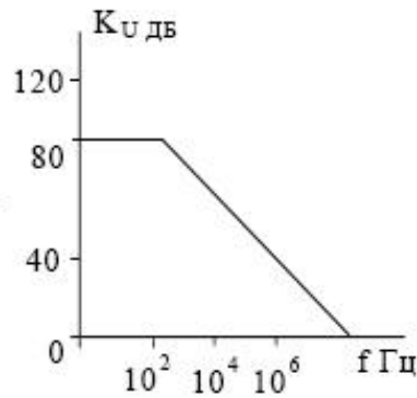
К140УД11
