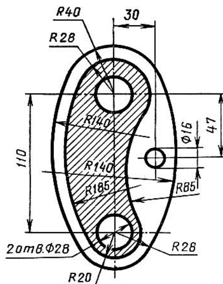
Коромысло
