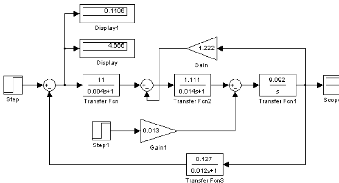
Рис. 2.15. ССДМ нескорректированного контура скорости
